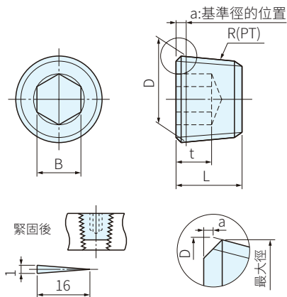
螺牙部 JIS B0203 R(PT)
